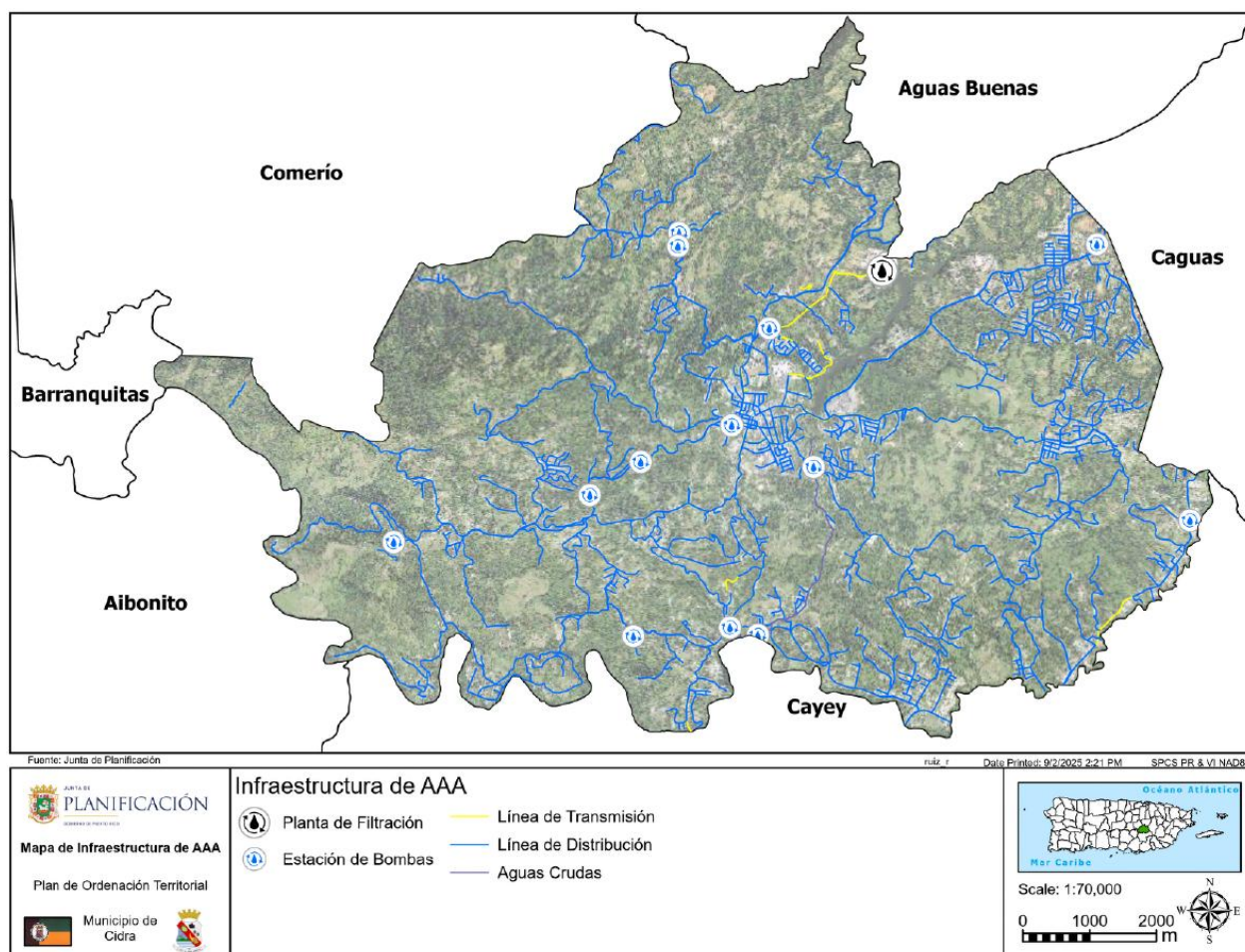
Figura 23: Mapa de infraestructura de la AAA en el municipio de Cidra
