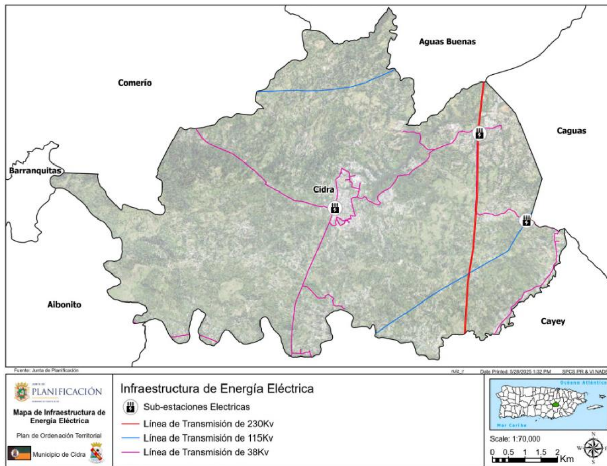
Figura 24: Sistema Eléctrico en el Municipio de Cidra
