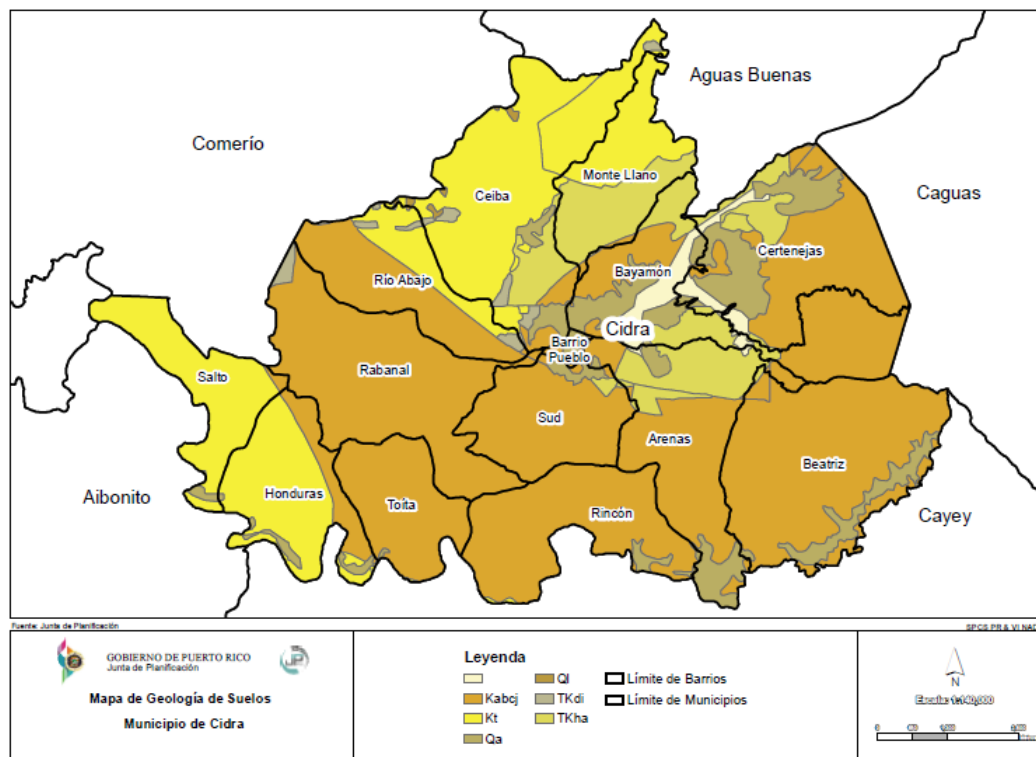
Figura 17. Mapa Geológico
